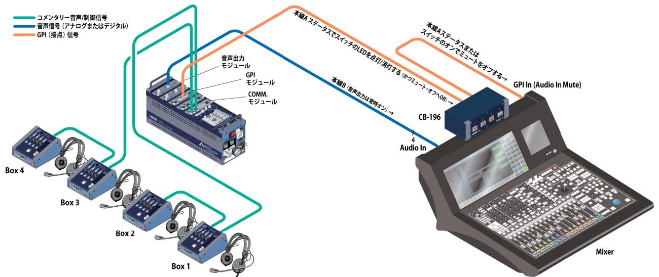
コメント音・ボックス本線の ON/OFF を外部 (ミキサー等) で行う場合
