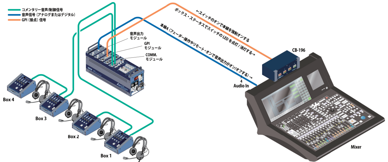
コメント音・ボックス本線の ON/OFF を LWB 内部で行う場合
